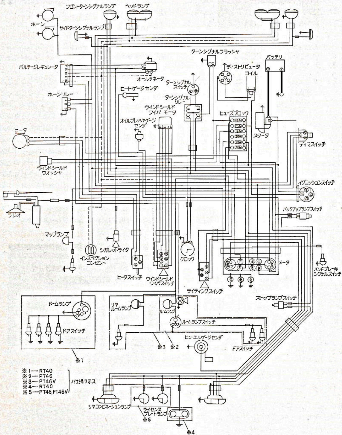
図5 電気結線関係図
